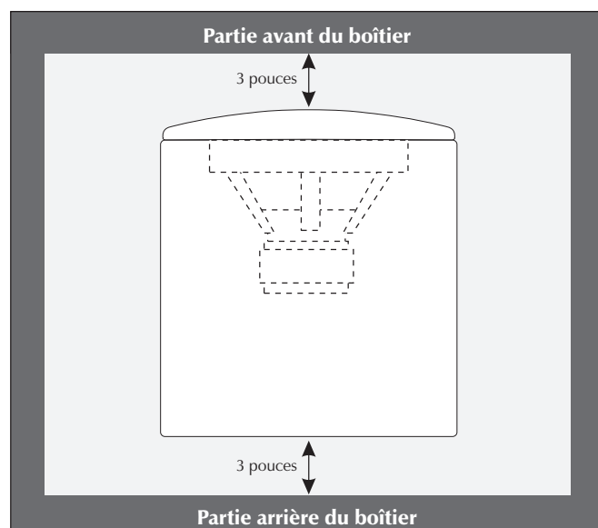
Figure 24. Lorsque le caisson de sous-graves est placé dans un boîtier, il faut un minimum de trois pouces d'espace libre à l'avant et à l'arrière.
